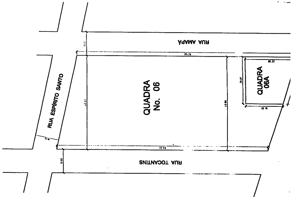
SITUAÇÃO EXISTENTE ESC 1 : 500
