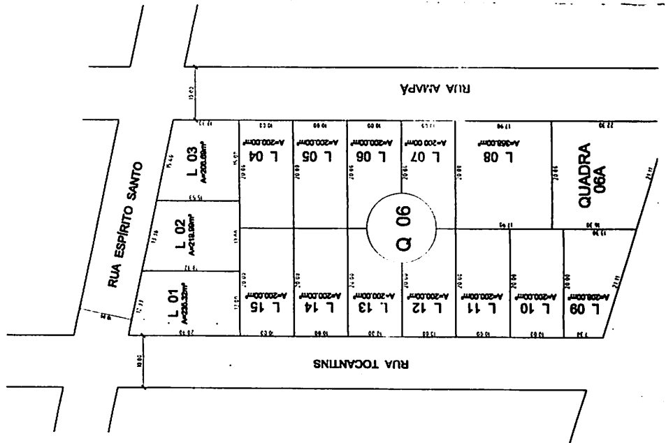
SITUAÇÃO PROPOSTA ESC 1 : 500
