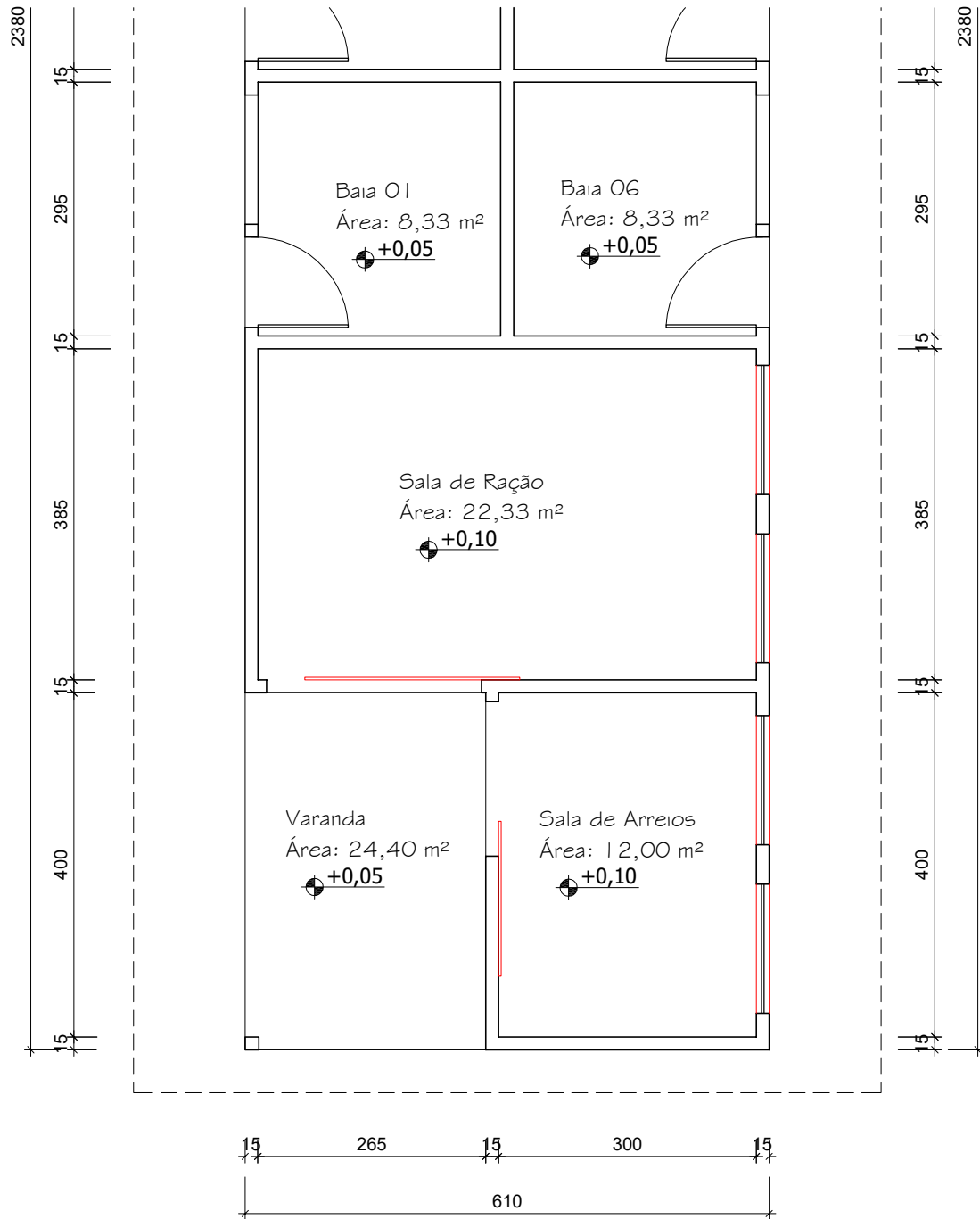
Planta Baixa - Baias Edificação 10 Área: 145,18 m 2 Escala 1:100
